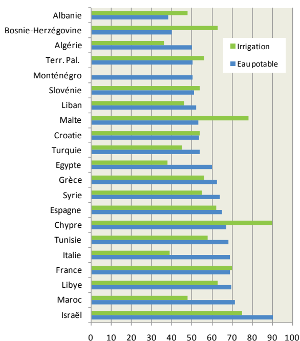
Figure 3 Efficience de l'utilisation de l'eau dans les deux secteurs en 2005 (%)
