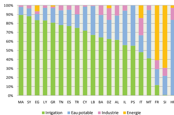
Figure 2 Demande totale en eau par secteur d'utilisation (période 2005-2007)
