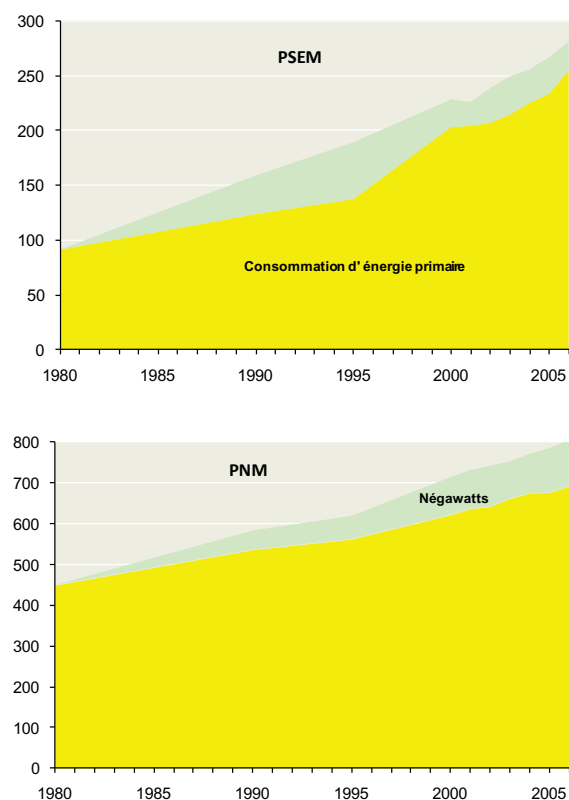
Figure 8 Potentiel des économies d'énergie à la baisse de l'intensité énergétique globale, 1980-2005 (Mtep)
