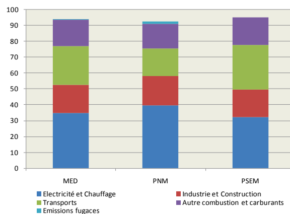
Figure 10 Répartition sectorielle des émissions de CO 2 issues de l'utilisation d'énergie par région depuis 1990 (%)
