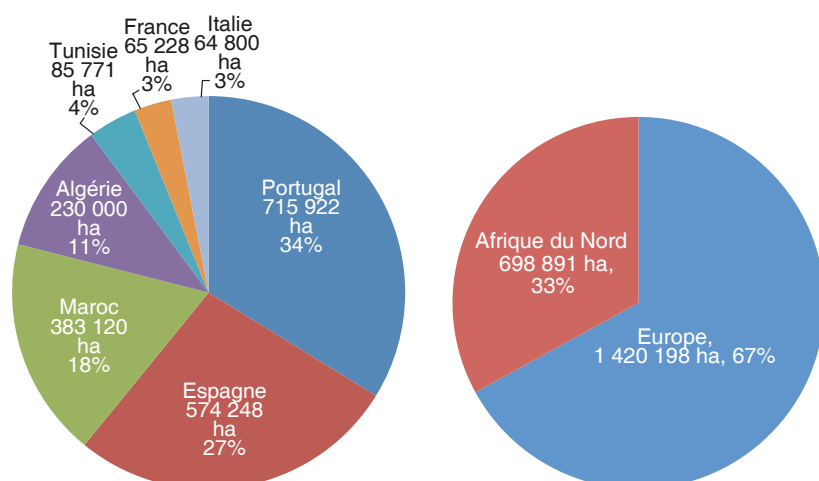
Figure 2.43. Surfaces des forêts de chênes liège et proportion de la surface nationale par rapport à l'ensemble de l'aire de répartition en 2012.
