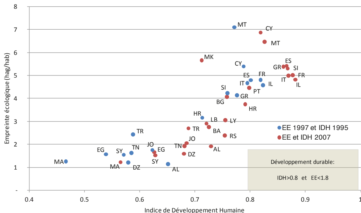
Figure 1.5. Comparaison entre les évolutions de l'Empreinte écologique (EE) et de l'Indice de Développement Humain (IDH) dans la région méditerranéenne, 2007.
