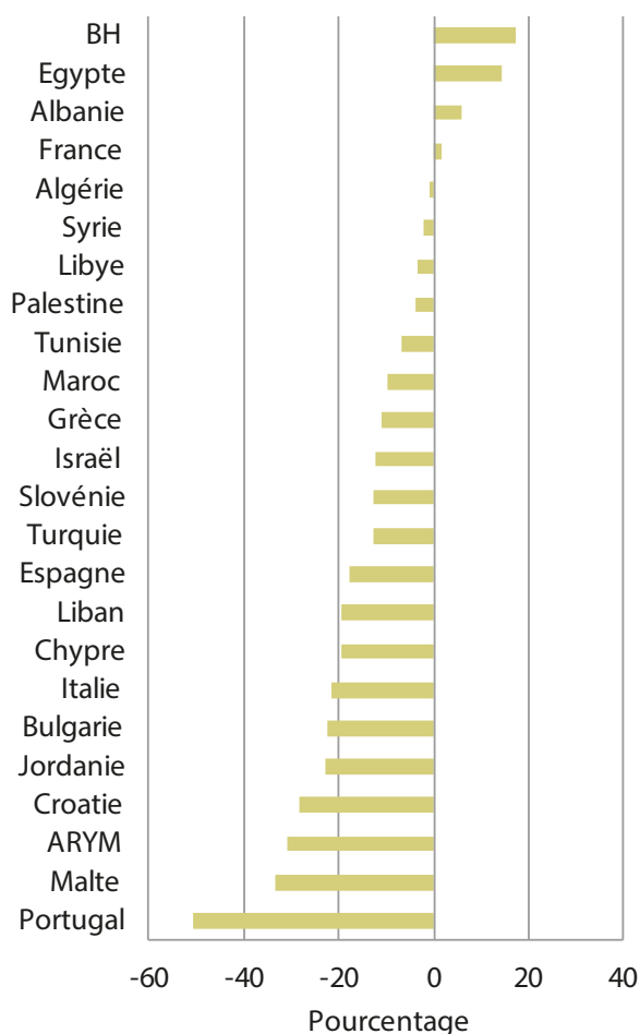
Figure 1.24. Perte nette de terres arables entre 1992 et 2009 (en pourcentage).
