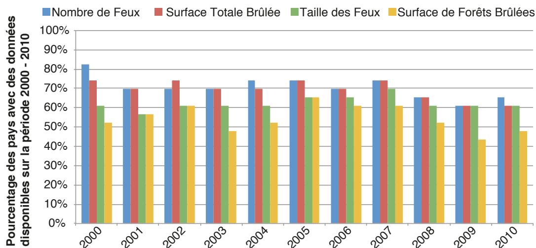
Figure 2.18. Disponibilité des données pour plusieurs variables sur les feux de forêts entre 2000 et 2010.
