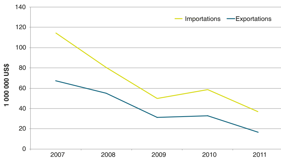
Figure 2.48. Evolution des importations et des exportations de produits en liège entre 2007 et 2011. Source : United Nations International Merchandise Trade Statistics, 2011.
