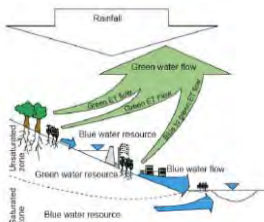
Figure 2.64. Flux des ressources en eau verte et en eau bleue.
