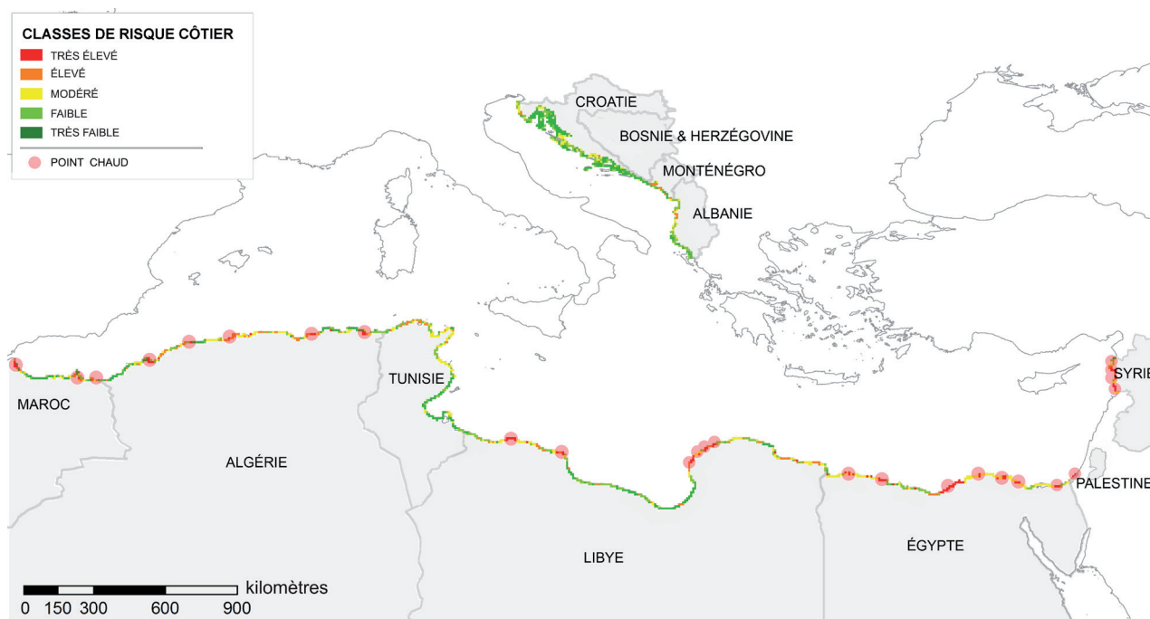
Figure 3 : Carte d'évaluation du risque régional basée sur la méthode CRI-MED
