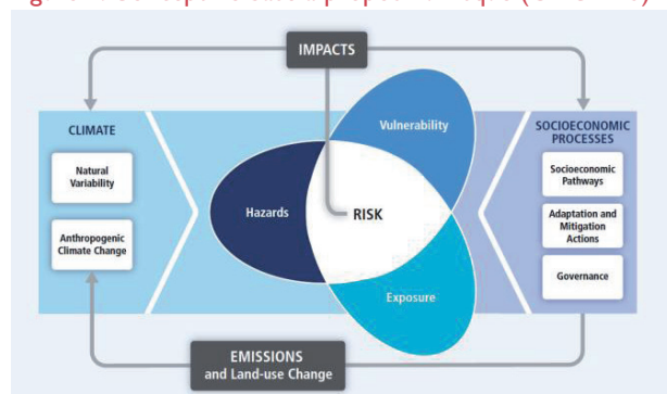
Figure 1: Concept de base à propos du risque (GIEC AR5)
